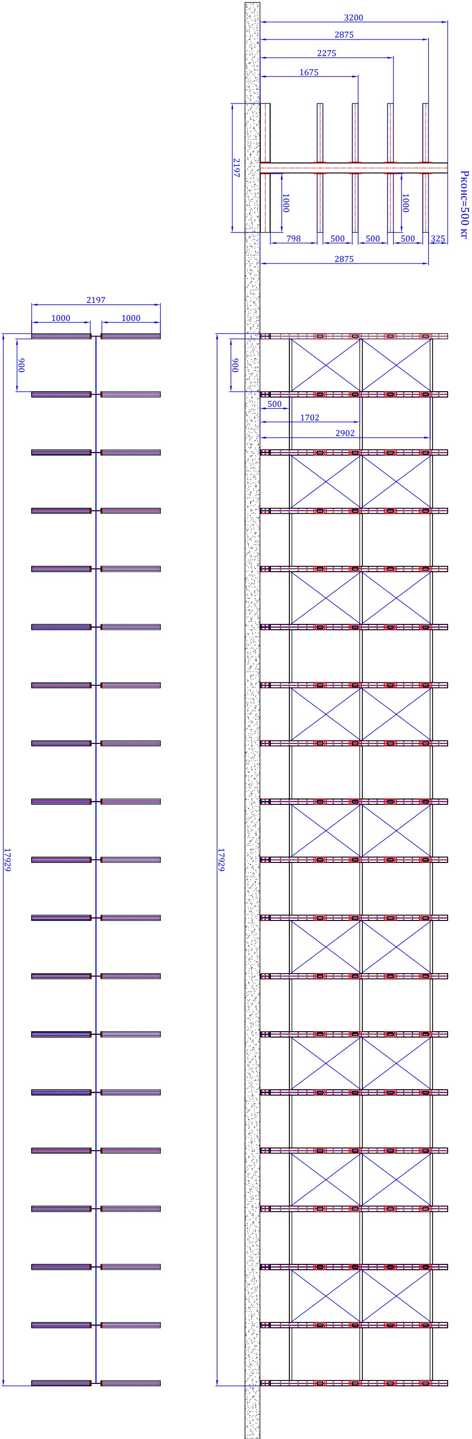
3. Стеллаж консольный двусторонний СК_17929х1187х3200_С19_К8-500-1000_1 шт
