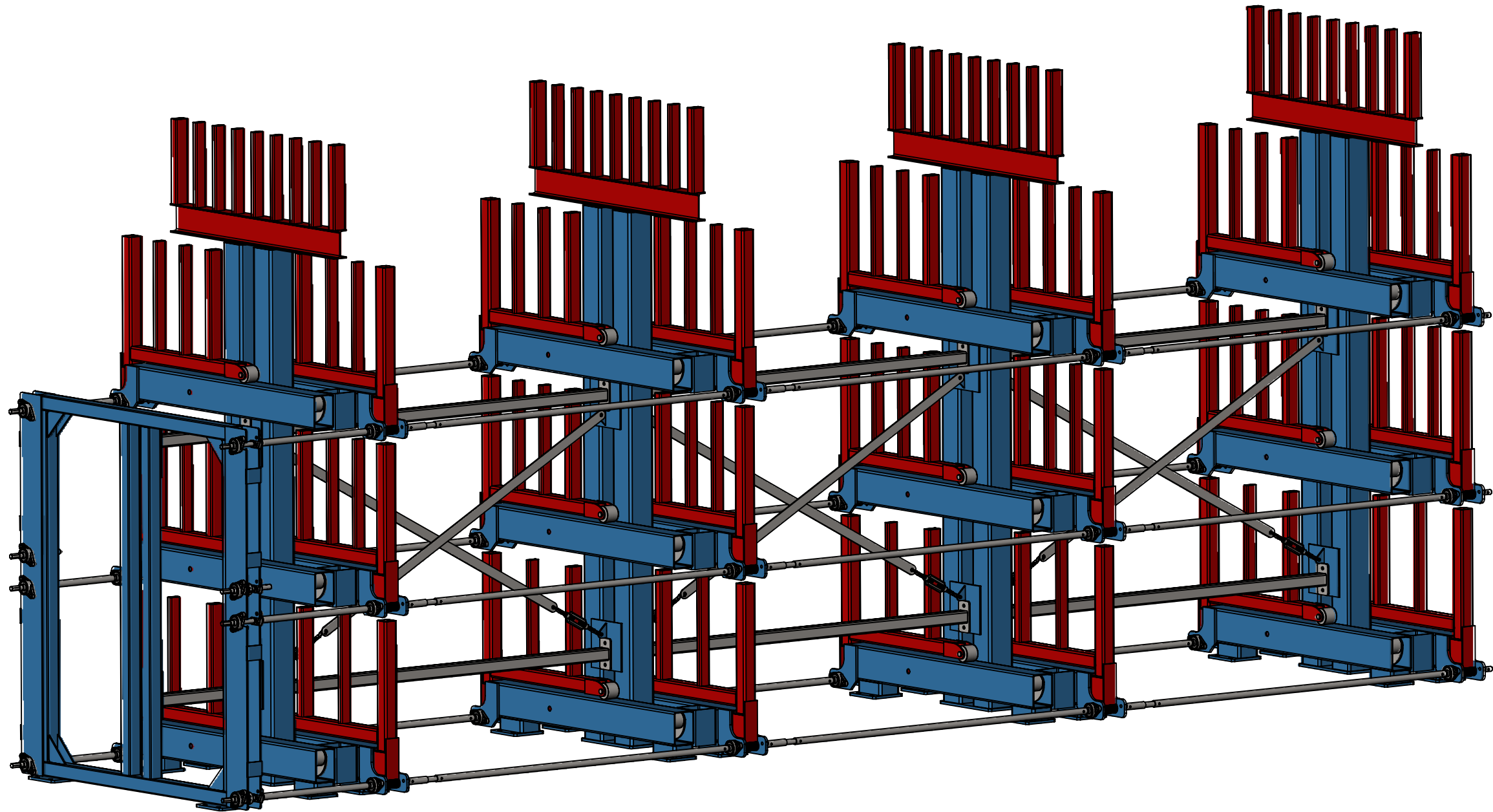
T25-180-3 СтВк 2-й 2х6 2м 3+1 Стеллаж с выдвижными консолями.
